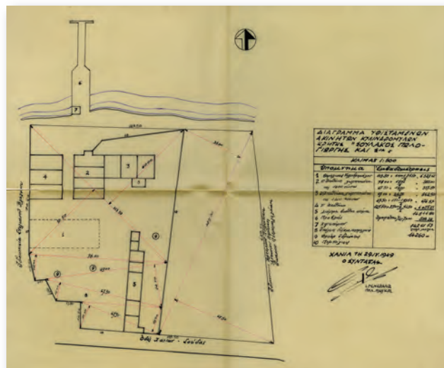
66. Διάγραμμα των εγκαταστάσεων των Κυλινδρόμυλων Κρήτης Σουλάκος Πωλογιώργης και Σία. Χανιά, 29 Απριλίου 1949.
