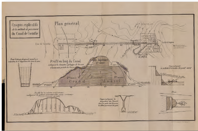
Σχέδιο για τη διάνοιξη του Ισθμού της Κορίνθου, Αθήνα 1883.
